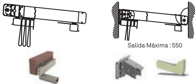
Fijación Lateral
